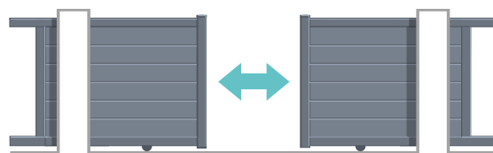
Portail coulissant double refoulement (uniquement sur ligne Active et série Ferronne)
